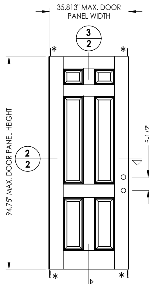
41 DOOR PANEL
